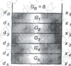
Рисунок 14.2. Набор сит с размерами ячеек d : d_1 = 3 \text{ мм} ; d_2 = 2 \text{ мм} ; d_3 = 1 \text{ мм} ; d_4 = 0,5 \text{ мм} ; d_5 = 0 .
