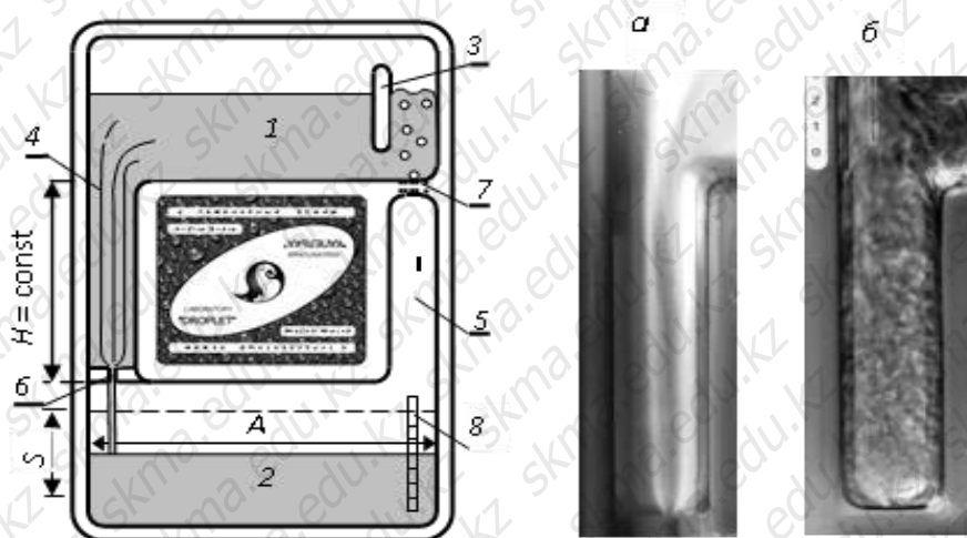
1, 2 – баки; 3 – перегородка; 4, 5 – опытные каналы; 6 – щель; 7 – решетка; 8 – равномерная шкала
