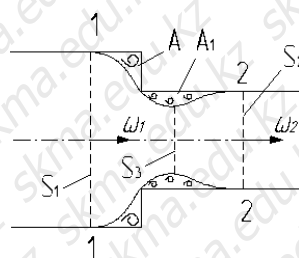
Рисунок 2- Внезапное сужение
