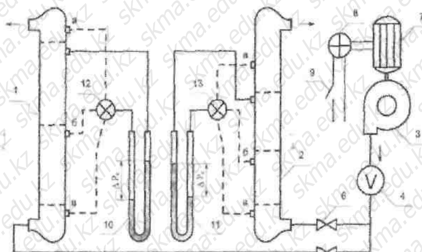
Рисунок 9.4. Схема экспериментальной установки
