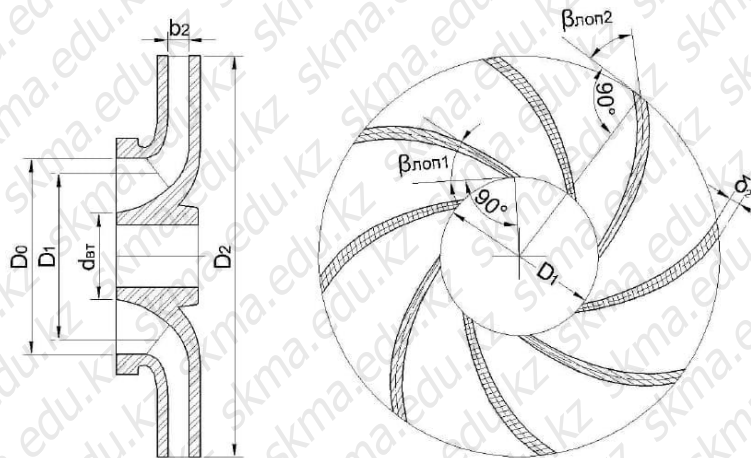
Рисунок 4. Эскиз рабочего колеса
